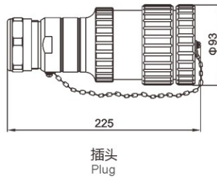
BLJ85-100、BLJ85-125
