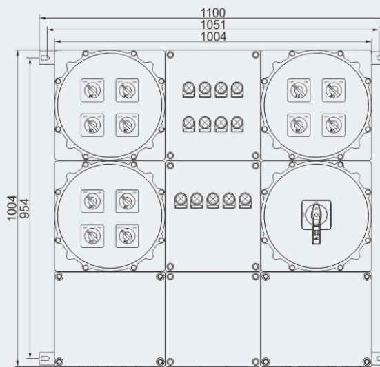
BXM(D)53-12/□/K/□
